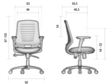
Silla operativa Cadeira operativa / Siège d'operative / Task chair / Drehsessel Stuhl.
